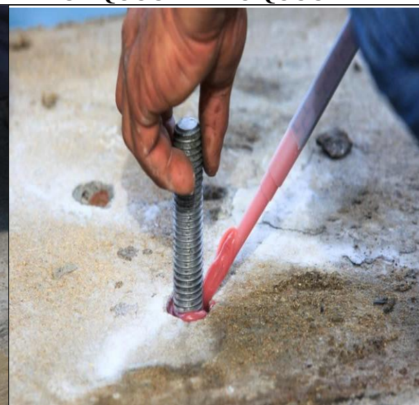
KHOAN CÂY THÉP ĐIỆN MẶT TRỜI ÁP MÁI NHÀ MÁY WAGON - KCN NHƠN TRẠCH III
