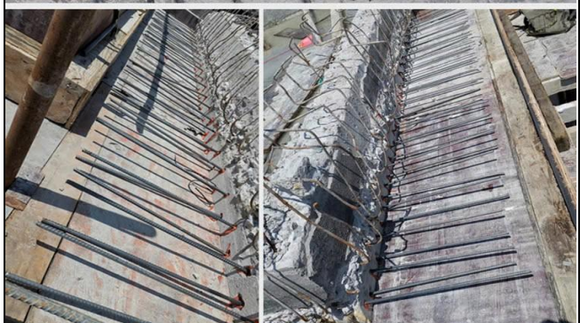
KHOAN CÂY THÉP BỂ LÀM MÁT- GÓI A1- LỘC HOÁ DẦU LONG SƠN
