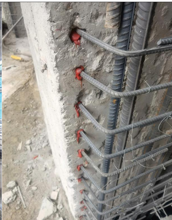
KHOAN CÂY THÉP NHÀ ĐIỀU HÀNH CẢNG HIDRO CARBON - LỘC HOÁ DẦU LONG SƠN
