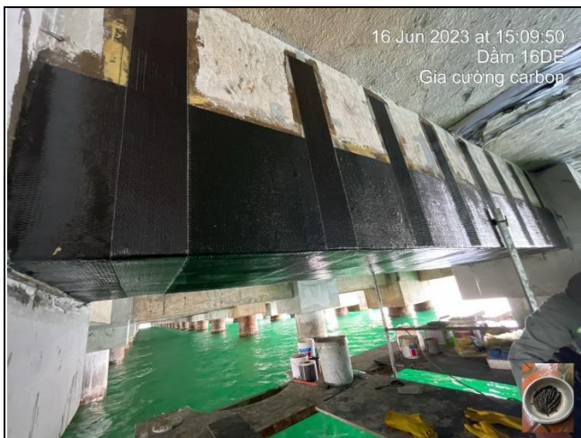
GIA CỐ KẾT CẤU CẦU CẢNG – PHÚ QUỐC
