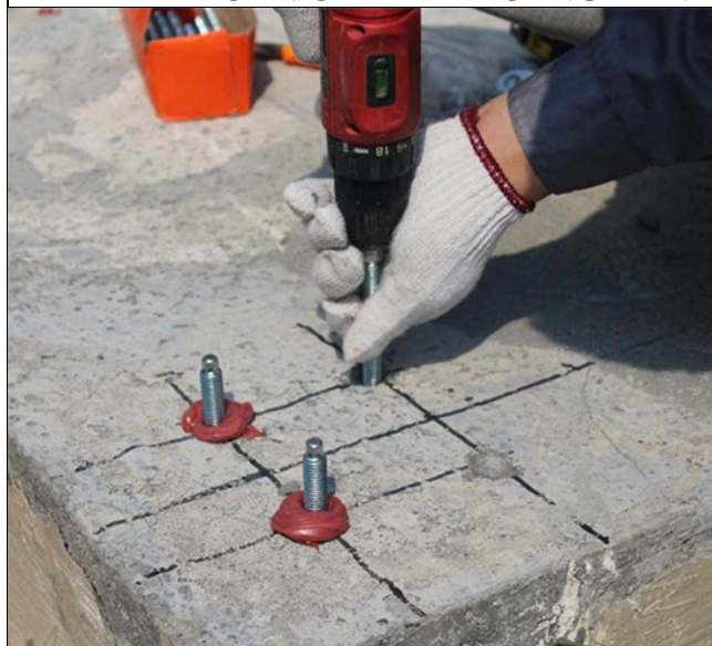
KHOAN CÂY THÉP ĐIỆN MẶT TRỜI ÁP MÁI NHÀ MÁY WAGON - KCN NHƠN TRẠCH III
