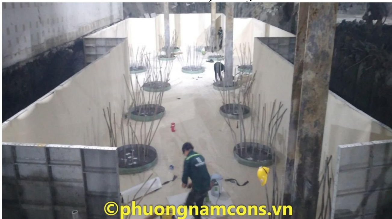
CHỐNG THÂM MÓNG – ĐIỆN GIÓ BẠC LIÊU
