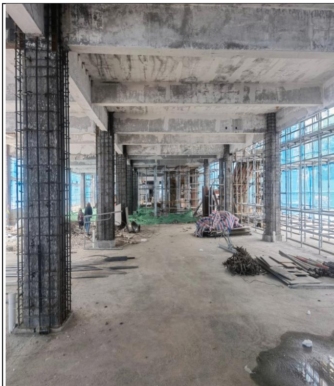
KHOAN CÂY THÉP NHÀ ĐIỀU HÀNH CẢNG HIDRO CARBON - LỘC HOÁ DẦU LONG SƠN
